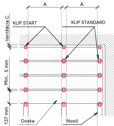
Obr. 4 Minimálne škáry medzi doskami a medzi doskami a pevným múrom
